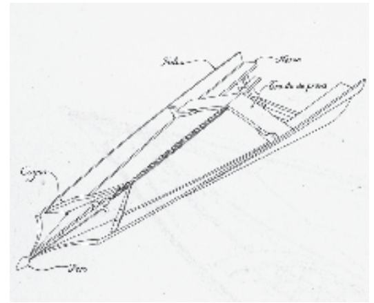
Nomenclatura dei componenti della parte prodiera del Puparin [tratto da «Le barche di Venezia, L'Altra Riva, 1981, di Ugo Pizzarello]
