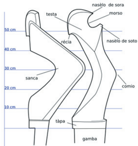
forcola: disegno schematico e nomenclatura [tratto da wikipedia.org]
