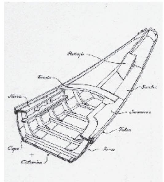
Nomenclatura dei componenti della parte poppiera del Puparin [tratto da «Le barche di Venezia, L'Altra Riva, 1981, di Ugo Pizzarello]
